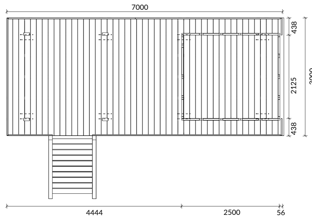
VISTA SUPERIOR
