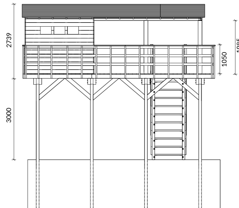
ALÇADO
